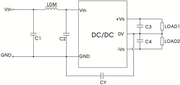
图 4.1 (其他输入推荐电路)
