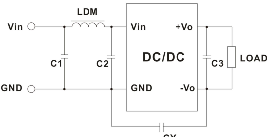
图 4.2 (5V 输入推荐电路)
