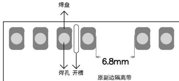
CLS05-15B12R3 推荐焊盘
