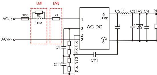
推荐电路 1
