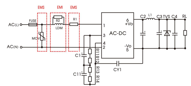
推荐电路 4
