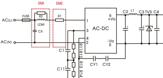
推荐电路 2
