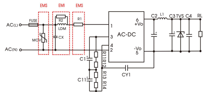
推荐电路 3
