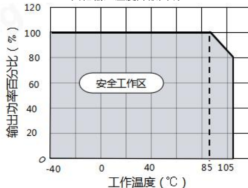
其他输入温度降额曲线 (b)
