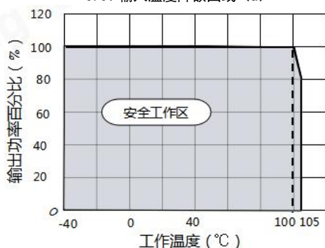
3.3V 输入温度降额曲线 (a)
