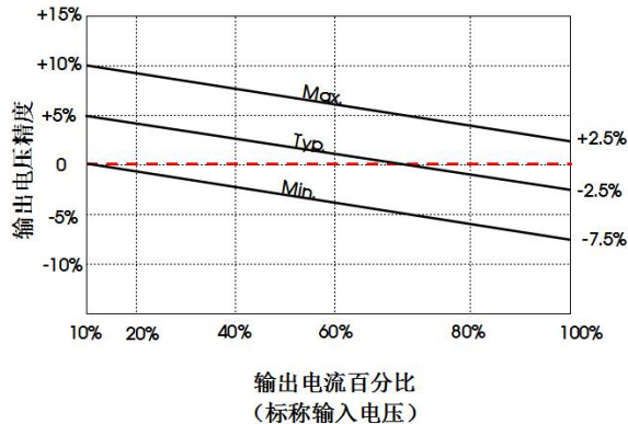
3.3/5VDC 输入其它输出 误差包络曲线图
