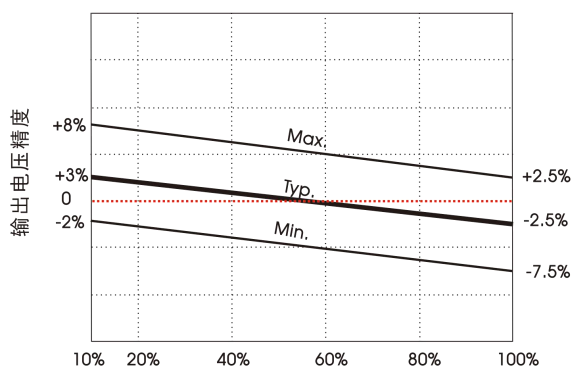
误差包络曲线图
