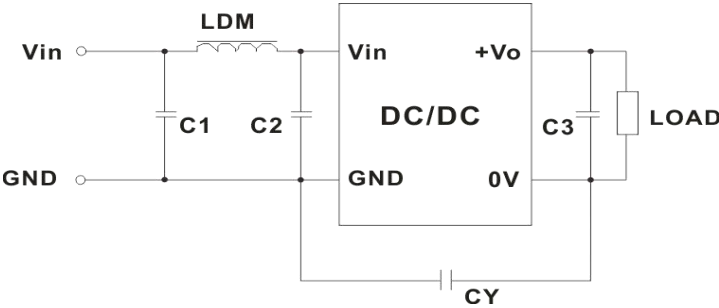
EMC 推荐电路参数值表
