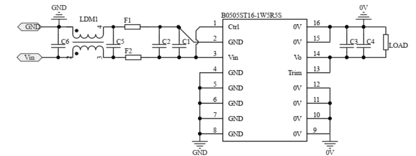
图3 CLASS A 推荐 EMI 外围
