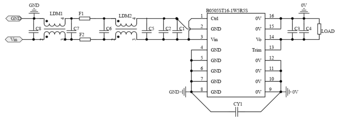
图4 CLASS B 推荐 EMI 外围
