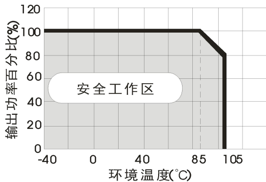
3.3V 输入 温度降额曲线图
