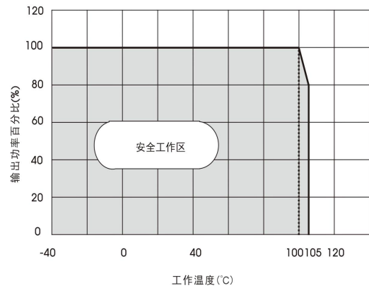
其他输入 温度降额曲线
