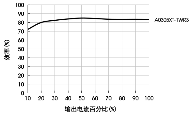
效率Vs输出负载 (Vin=3.3V)
