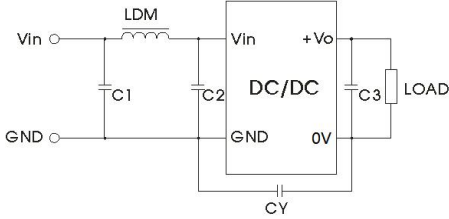
正负双路
