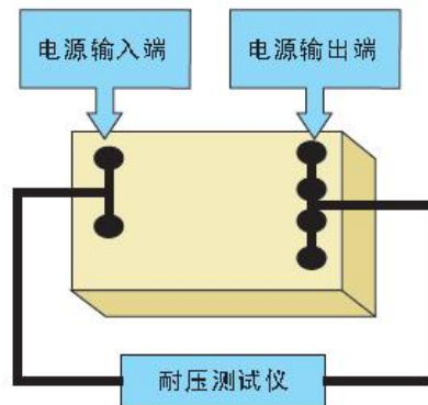
图 4-5 耐压测试图
