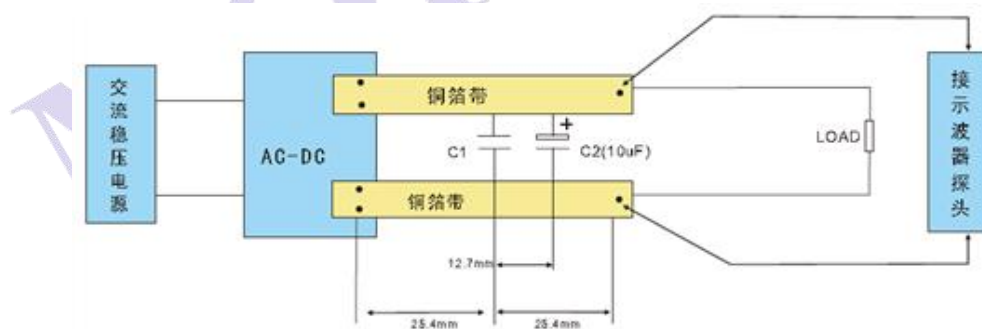
图 4-1 平行线测试法
