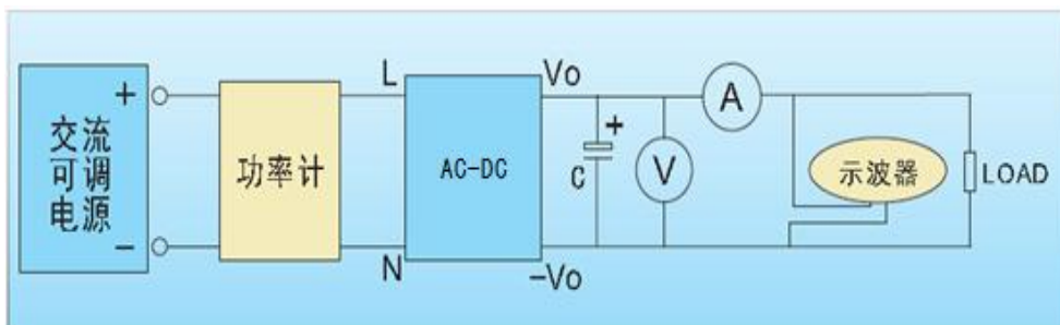
图 3-1 基本测试电路连接
