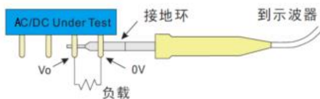
图 4-3 靠测法
