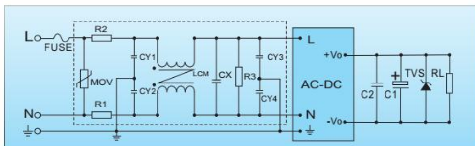
图 3-3 典型输入 EMC 滤波电路
