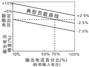
误差包络曲线图
