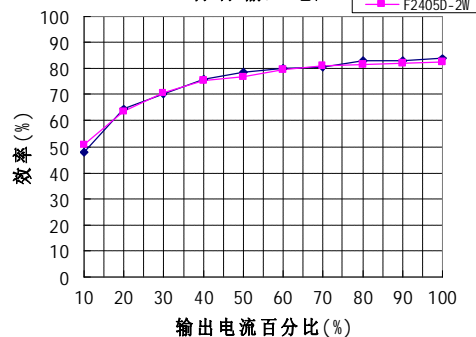
输出负载VS效率曲线图
