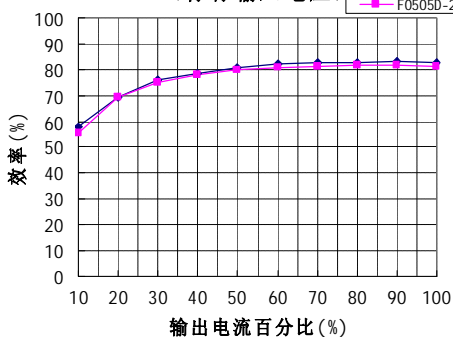
输出负载VS效率曲线图
