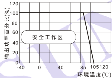
温度曲线图
