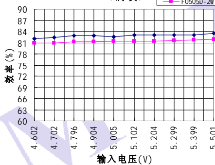
输入电压VS效率曲线图
