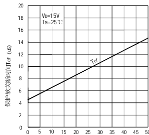
外接 C f 的取值 (pF) (PIN: 10-14)
