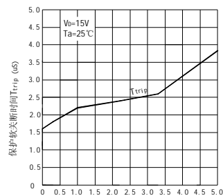
外接 C trip 的取值 (nF) (PIN: 12-16)
