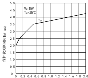
外接 R f 的取值 (K \Omega ) (PIN: 14-15)
